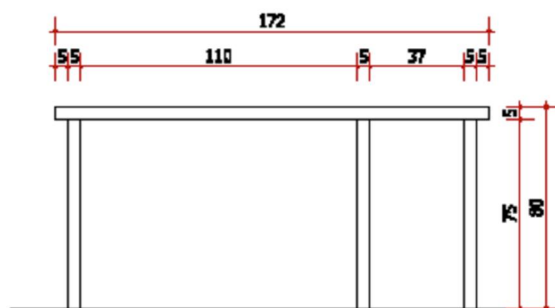
PRESEK 1-1
