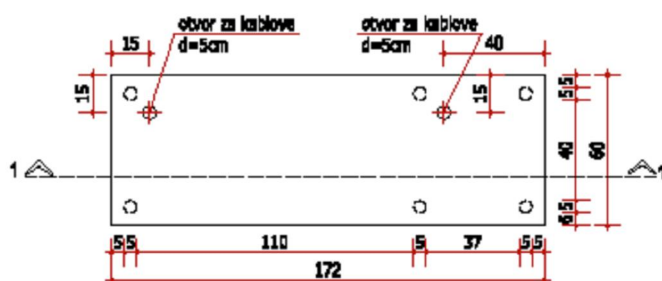
POGLED A
