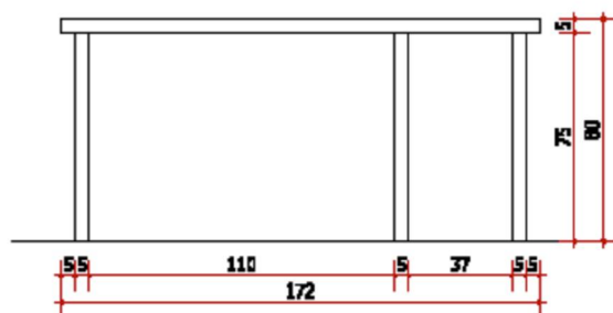
POGLED A
