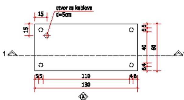
POGLED A
